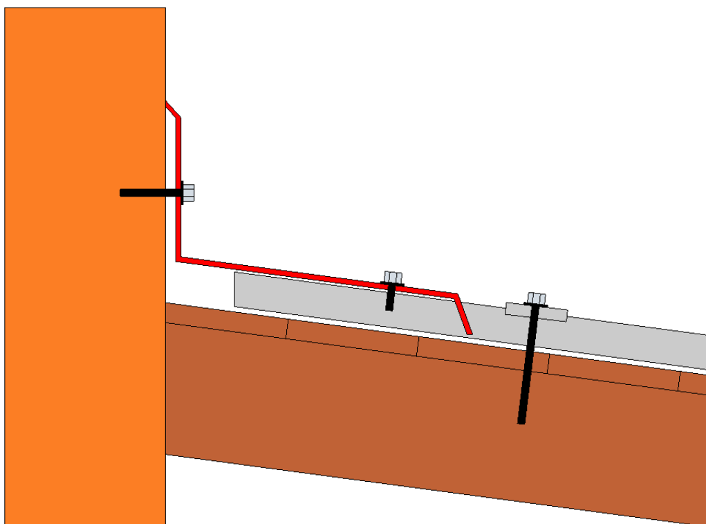
Výkres 8: Lišta ke zdi čelní – horní
