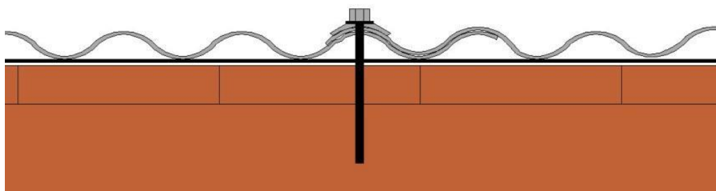
Překrytí v krajní vlně a kotvení šroubem a kalotou přes vodní drážku
