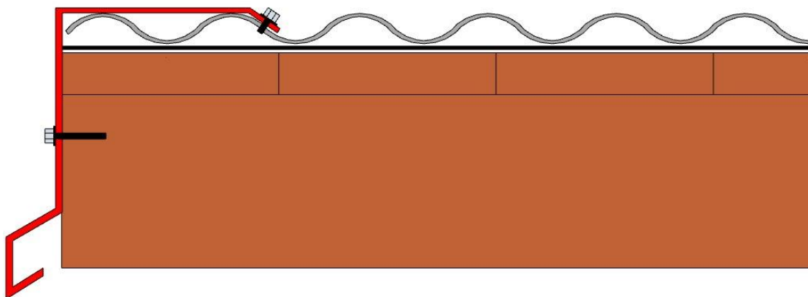
Výkres 7: Závětrná lišta
