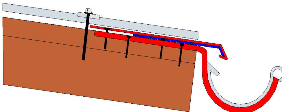
Výkres 1: Detail odkapní hrany
