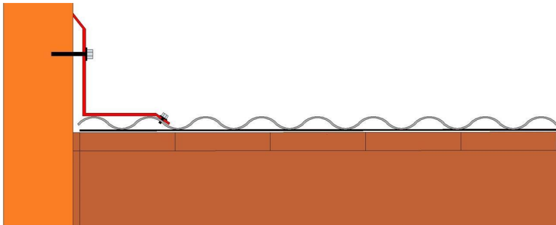
Výkres 6: Boční lišta
